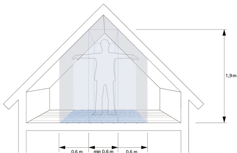
§ 6-1 Figur 1: Måleverdige gulvplan på loft.
