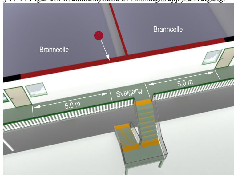
1) Branncellebegrensende vegg mot svalgangen.
