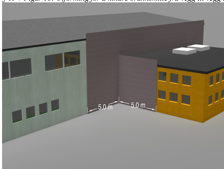
§ 11-7 Figur 1b: Utforming for å hindre brannsmitte fra vegg til vegg i innvendige hjørner.
